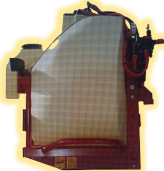
Cuve Physeter 750 litres Hauteur 1200 x largeur 2000 x prof 850 mm
